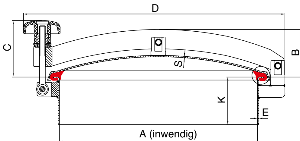
Afdichtingsdetail NW 200-800
